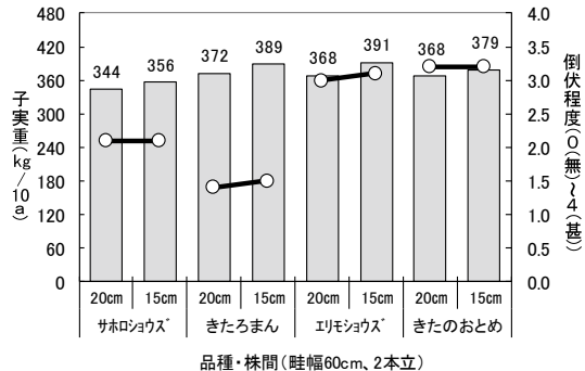
図9-15 早・中生小豆栽植密度試験 (十勝農試、平成13～16年)
