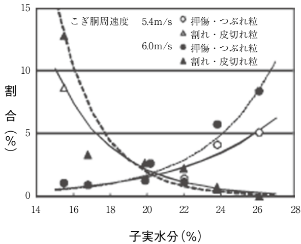
図 12-12 子実水分と損傷粒割合
