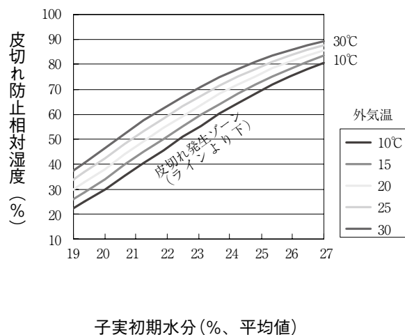
図12-16 常温通風乾燥における皮切れ防止相対湿度の下限值
