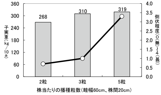
図9-13 「エリモショウス」 播種量試験 (十勝農試、平成10～12年)
