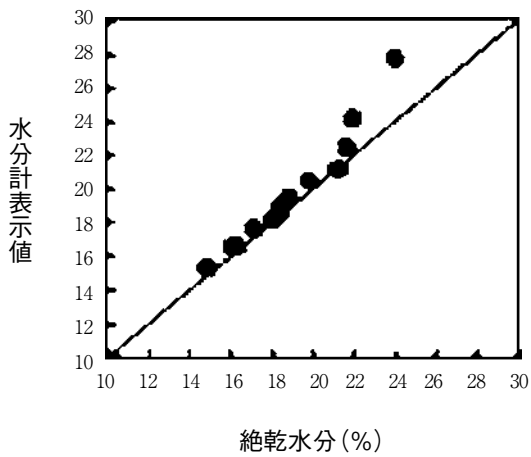
図 12-17 絶乾法による子実水分と簡易水分
