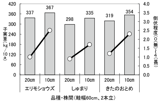
図9-14 中生小豆栽植密度試験 (十勝農試、平成8～11年)
