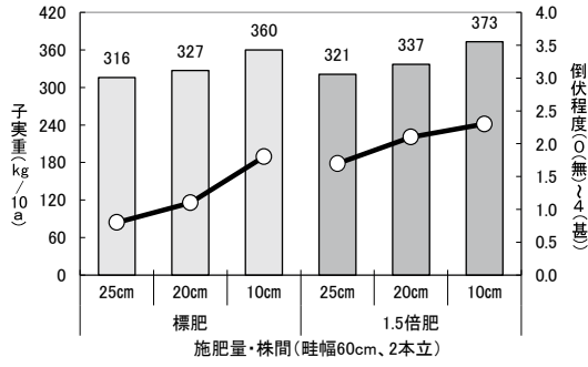
図9-12 「エリモショウス」 栽植密度試験 (十勝農試、平成7～9年)
