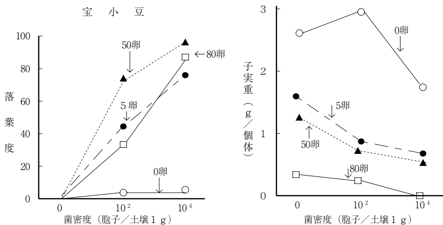
図 11-33 ダイズシストセンチュウおよび菌密度と発病または子実重との関係
