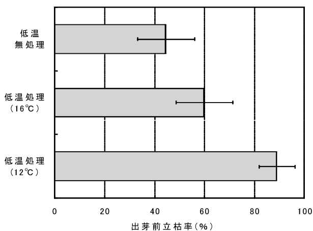
図 11-3 低温処理が連作土壌におけるダイズ苗立枯病の発病におよぼす影響
