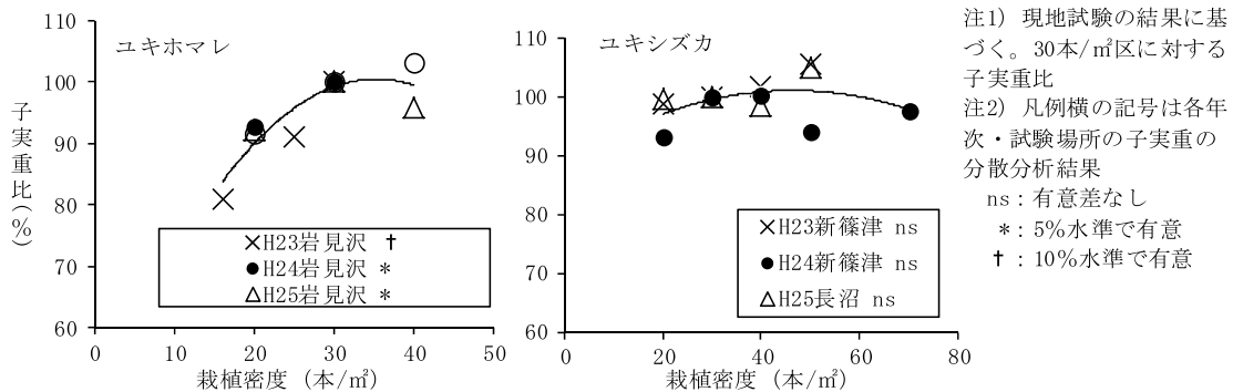
図9-10 狭畦栽培における栽植密度と子実重の関係
