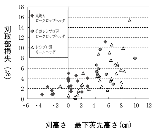
図12-7 豆用コンバインの刈取部損失
