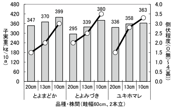
図9-6 十勝大豆栽植密度試験 (十勝農試、平成28～29年)
