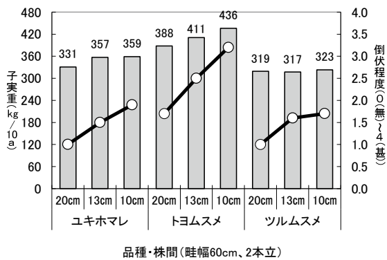
図 9-2 道央大豆栽植密度試験 (十勝農試、平成 11 ~ 13 年)
