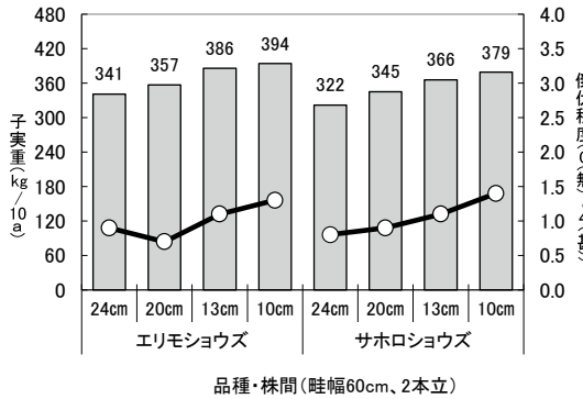
図9-16 網走小豆栽植密度試験 (北見農試、平成7～9年)
