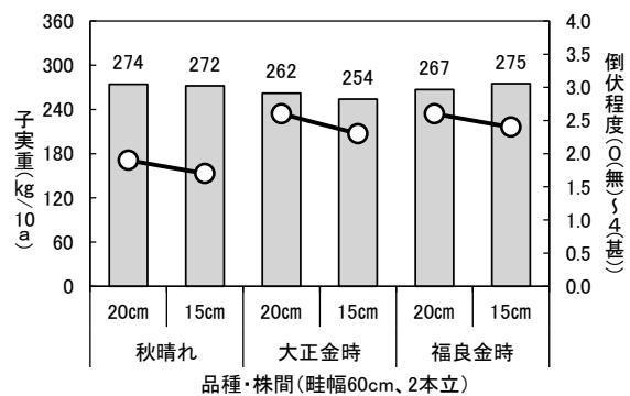
図9-23 金時栽植密度試験 (十勝農試、平成27～28年)
