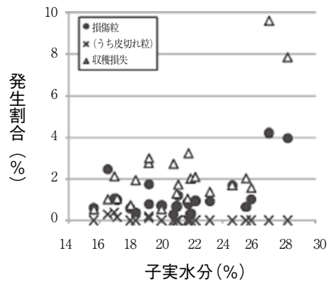
図 12-14 子実水分と収穫損失、損傷粒の割合
