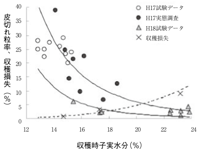
図12-5 黒大豆の収穫時子実水分と皮切れ粒率の関係
