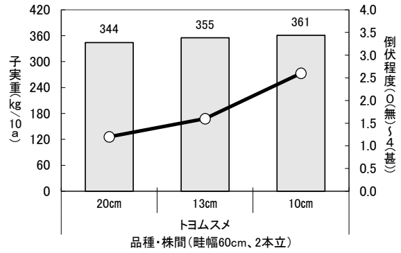
図9-7 十勝中生大豆栽植密度試験 (十勝農試、平成14～16年)
