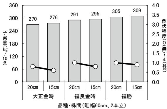
図9-20 金時栽植密度試験 (十勝農試、平成10～13年)
