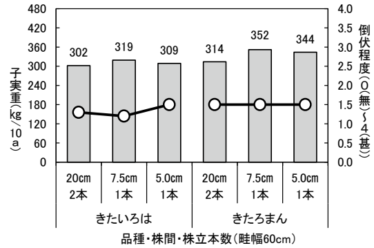
図9-19 小豆栽植密度試験 (十勝農試、令和2～4年)
