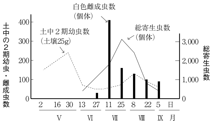
図 11-32 大豆におけるダイズシストセンチュウの発生長
