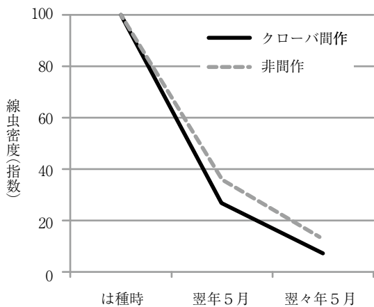
図 11-35 クローバ間作、非間作下の線虫推移 クローバは種時密度を 100 とした時の各調査時における密度指数
