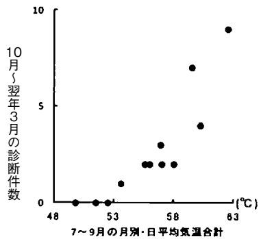
図 11-30 7～9月の温度と診断件数 (1999～2010年)
