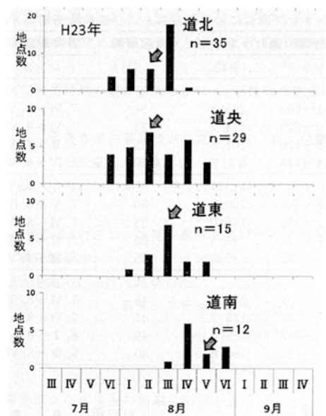
図 11-7 フェロモントラップ調査による成虫の誘殺最盛期の分布（平成 23 年）
