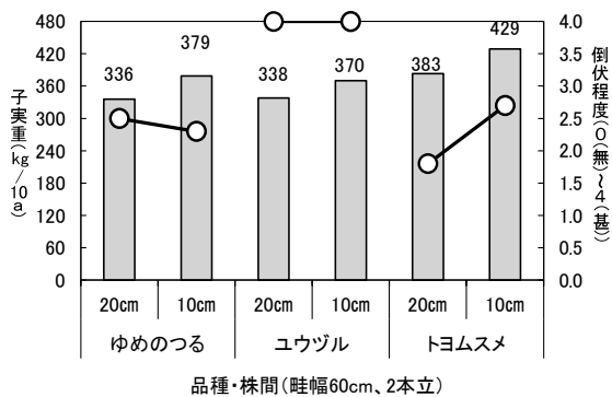
図 9-4 極大粒大豆栽植密度試験 (中央農試、平成 21 ~ 22 年)
