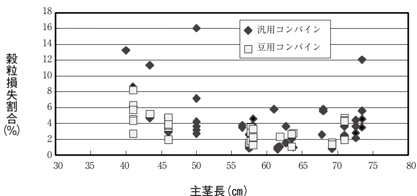
図12-1 主茎長と穀粒損失の割合
