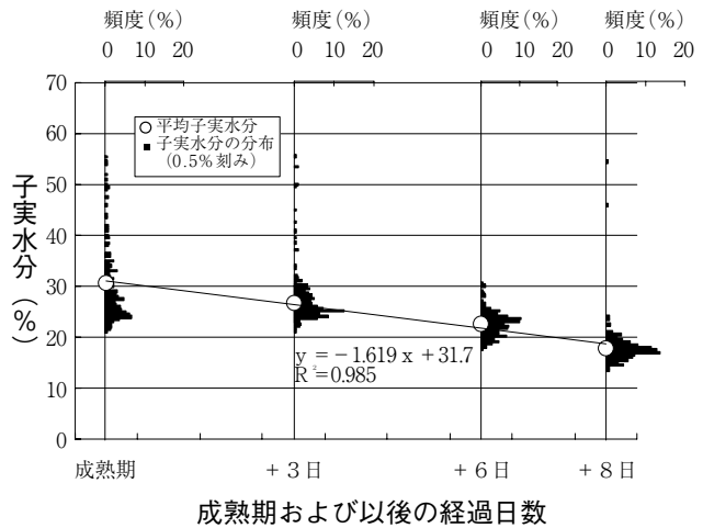
図 12-13 成熟期以降の子実水分の分布と平均
