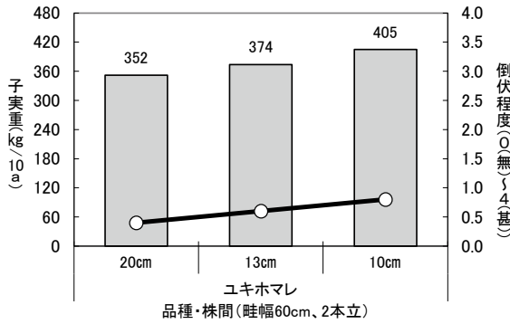
図9-8 網走早生大豆栽植密度試験 (北見農試、平成11～12年)
