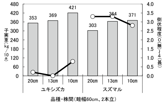
図9-9 納豆用大豆栽植密度試験 (十勝農試、平成12～13年)
