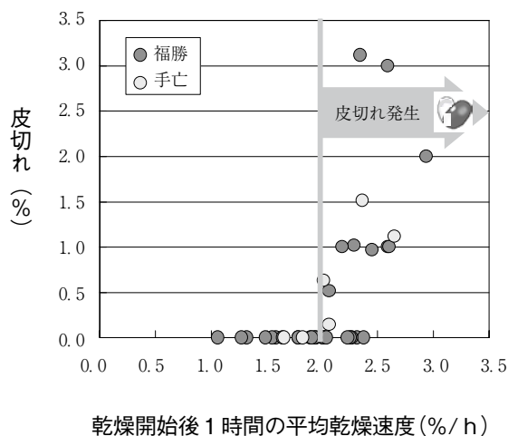
図12-15 乾燥開始後1時間の乾燥速度と皮切れ粒の発生条件
