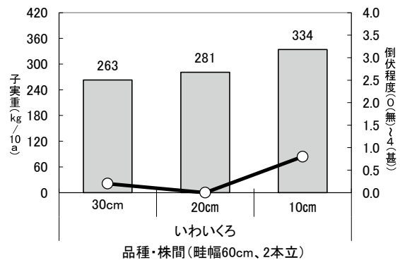
図 9-3 黒大豆栽植密度試験 (中央農試、平成 7 ~ 9 年)
