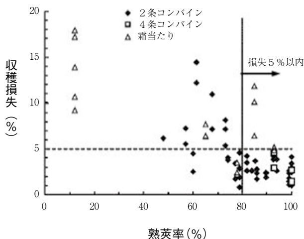
図 12-9 熟莢率と収穫損失
